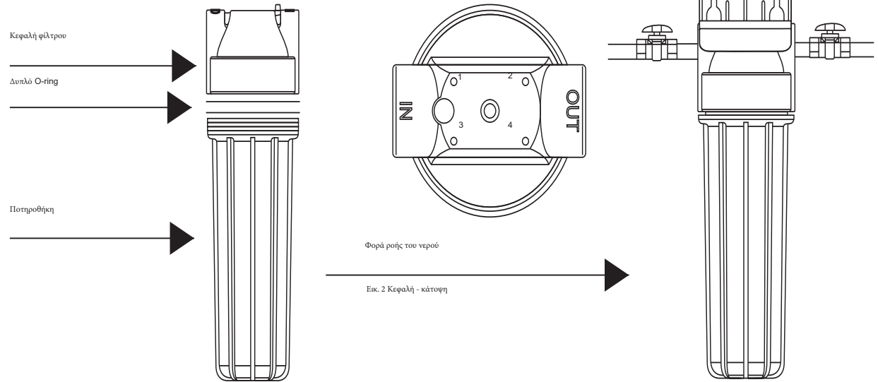
Εικ. 3 Έναιο φίλτρο κρύου νερού Είσοδος- Έξοδος εγκατάσταση
